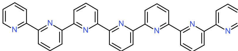
2,2':6',2'':6'',2''':6''',2''''':6''''',2''''''- Septipyridine
