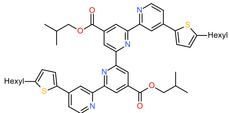
Di-isobutyl 4,4''-bis(5-hexyl-2-thienyl)- 2,2':6',2'':6'',2''':6''',2''''-Quaterpyridine]-4',4''- dicarboxylate
