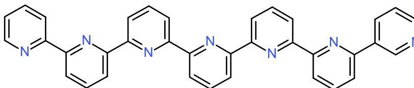
2,2':6',2'':6'',2''':6''',2''''':6''''',3''''''- Septipyridine
